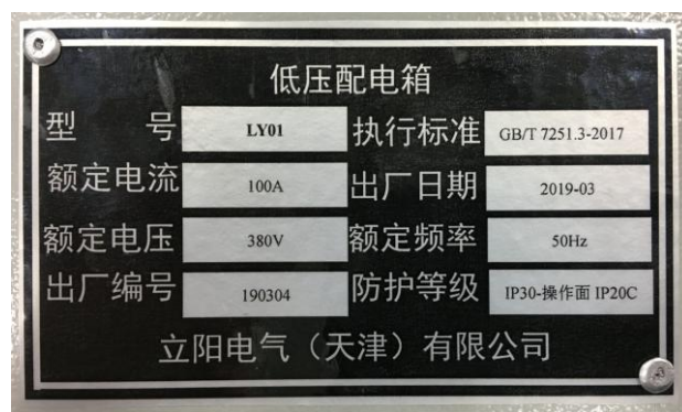
铭牌照片
