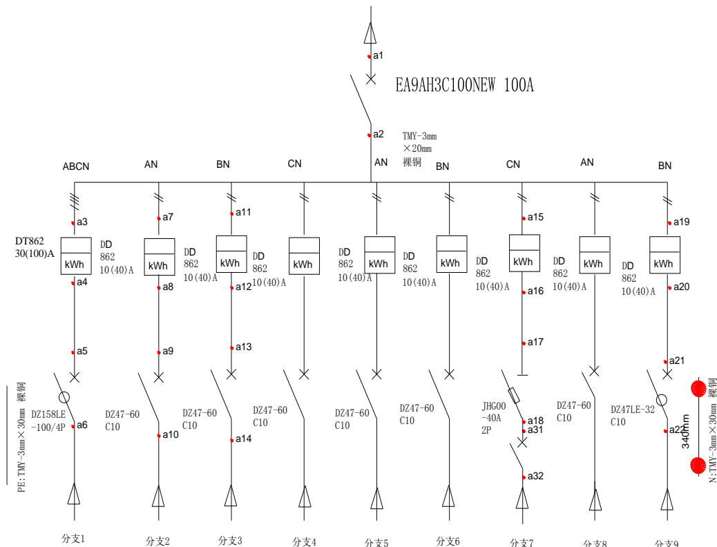
温升示意图 F1:
